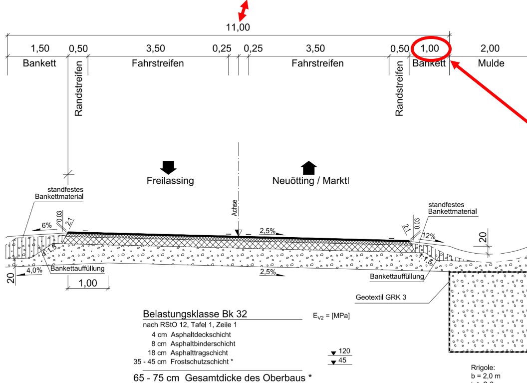
Bild 6: Regelquerschnitt RQ 11,5+
