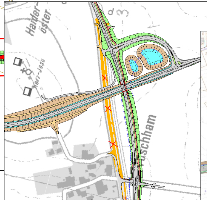
Vorentwurf M = 1:5.000
