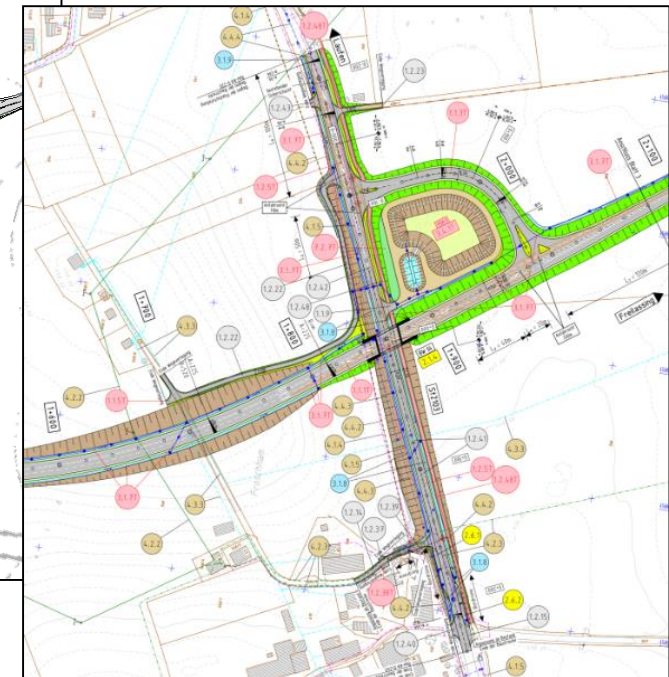
Planfeststellung M = 1:1.000
