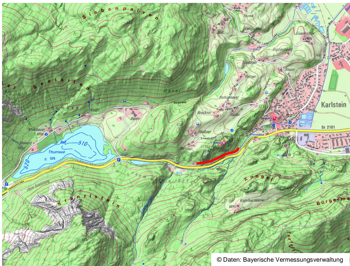
Lageplan Steinschlagschutzzaun
